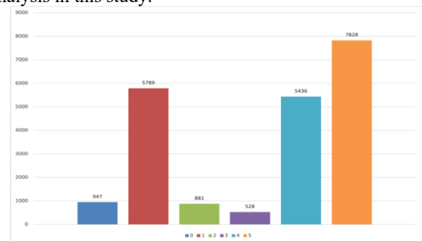
Fig. 2 – Data count.
