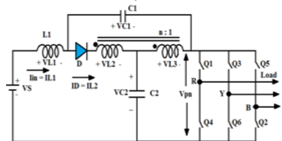
Fig. 2 – Trans-QZSI.
