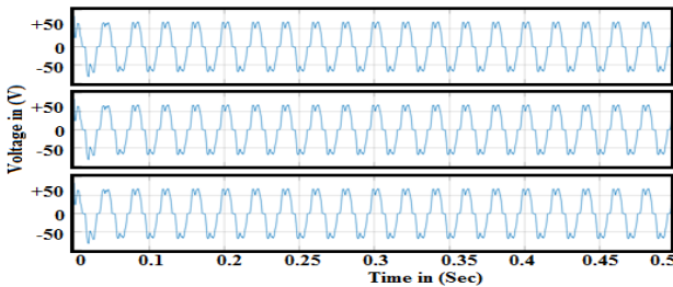
Fig. 7 – PMSG output voltage.
