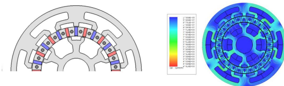
Fig. 12 – MVMP cu dublu stator în formă de poli crestați și magneți dispuși radial: stânga – structura motorului, dreapta – harta inducției magnetice la cuplu maxim [31].
