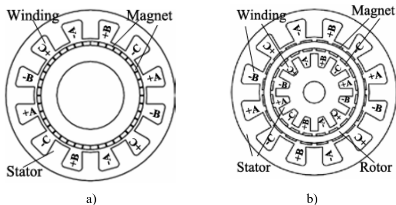
Fig. 10 – MVMP cu a) magnăți cu distribuție Halbach, b) cu dublu stator [27].
