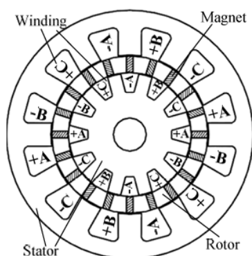
Fig. 9 – MVMP cu dublu stator și magneți dispuși radial (spîțe) [25].
