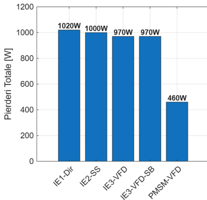
Fig. 4 – Pierderi totale.
