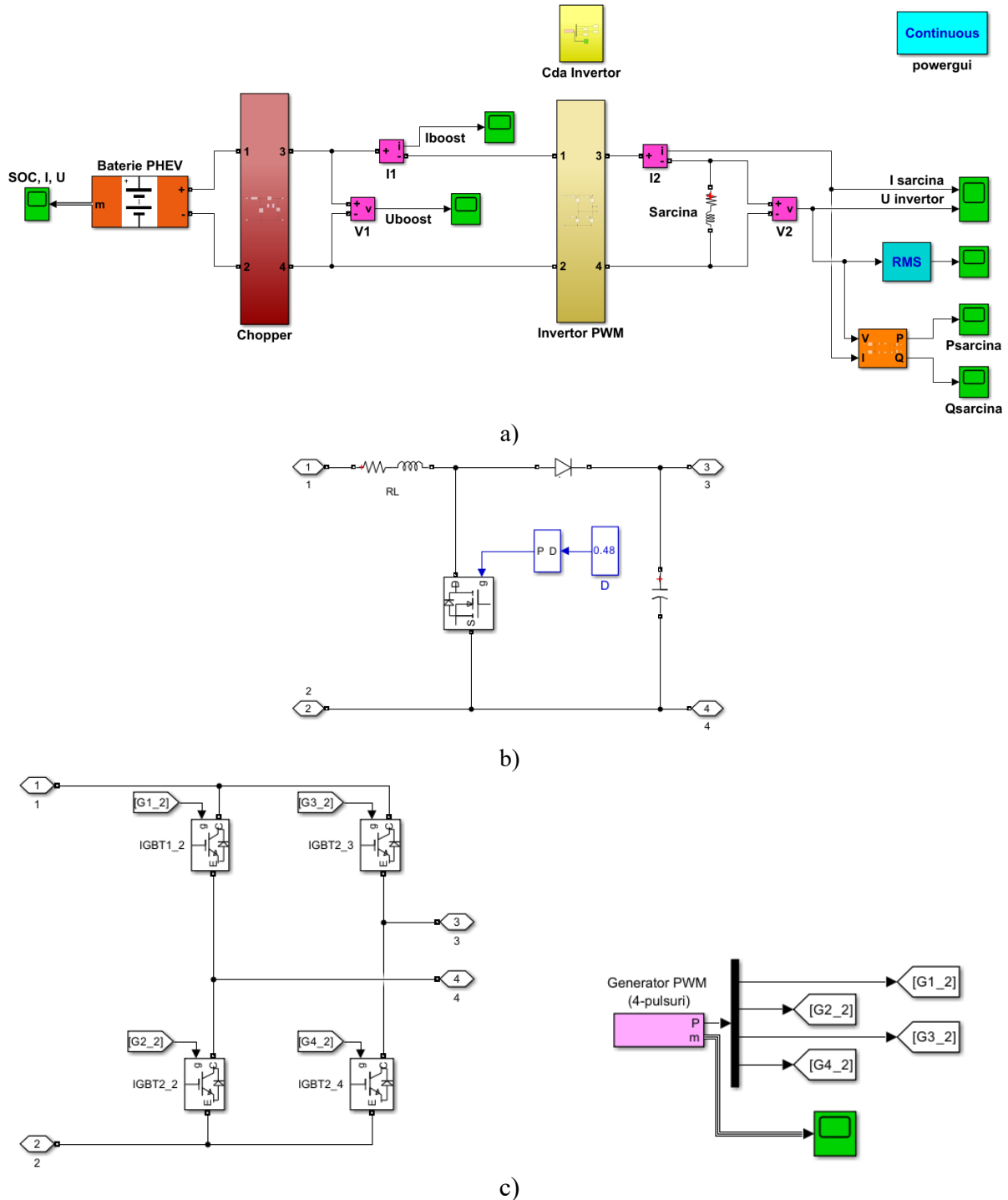
Fig. 3 – Schema bloc dezvoltată în Matlab/Simulink folosită în analiza numerică în scenariul V2L în care bateria PHEV alimentează o rețea de consumatori; a) schema de ansamblu; b) chopper ridicător; c) invertor PWM și comanda asociată.
