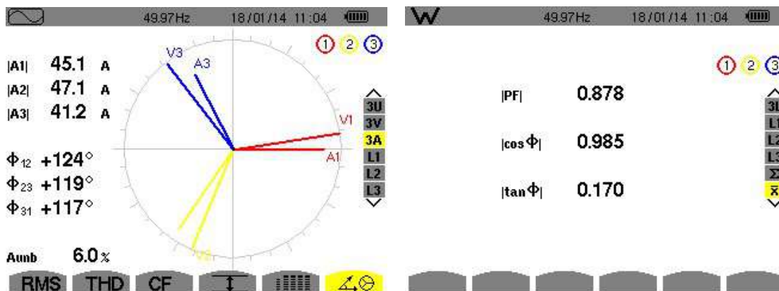
Fig. 7 Diagramele fazoriale ale armonicilor fundamentale pentru tensiunile și curenți de fază măsurati în secundar.
